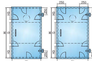
BF, CF型 TYPE BF, CF
