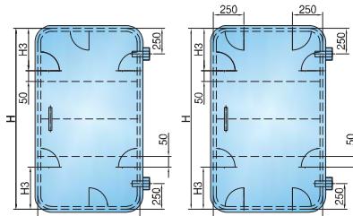
AY型 TYPE AY
