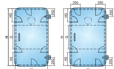
BY, CY型 TYPE BY, CY
